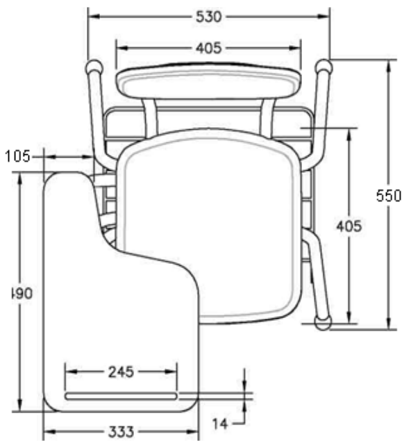
VISTA SUPERIOR
