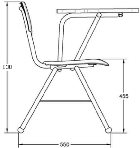
VISTA LATERAL
