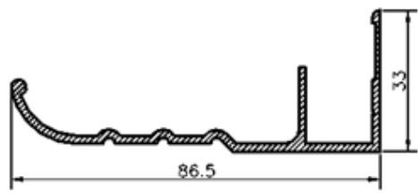
PORTA GIS
