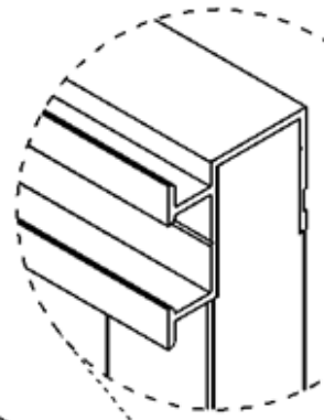
DETALLE DE CANAL SUPERIOR PARA CORCHO
