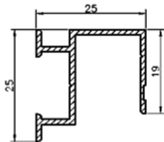
CANAL SUPERIOR
