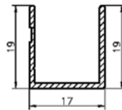
CANAL LATERAL
